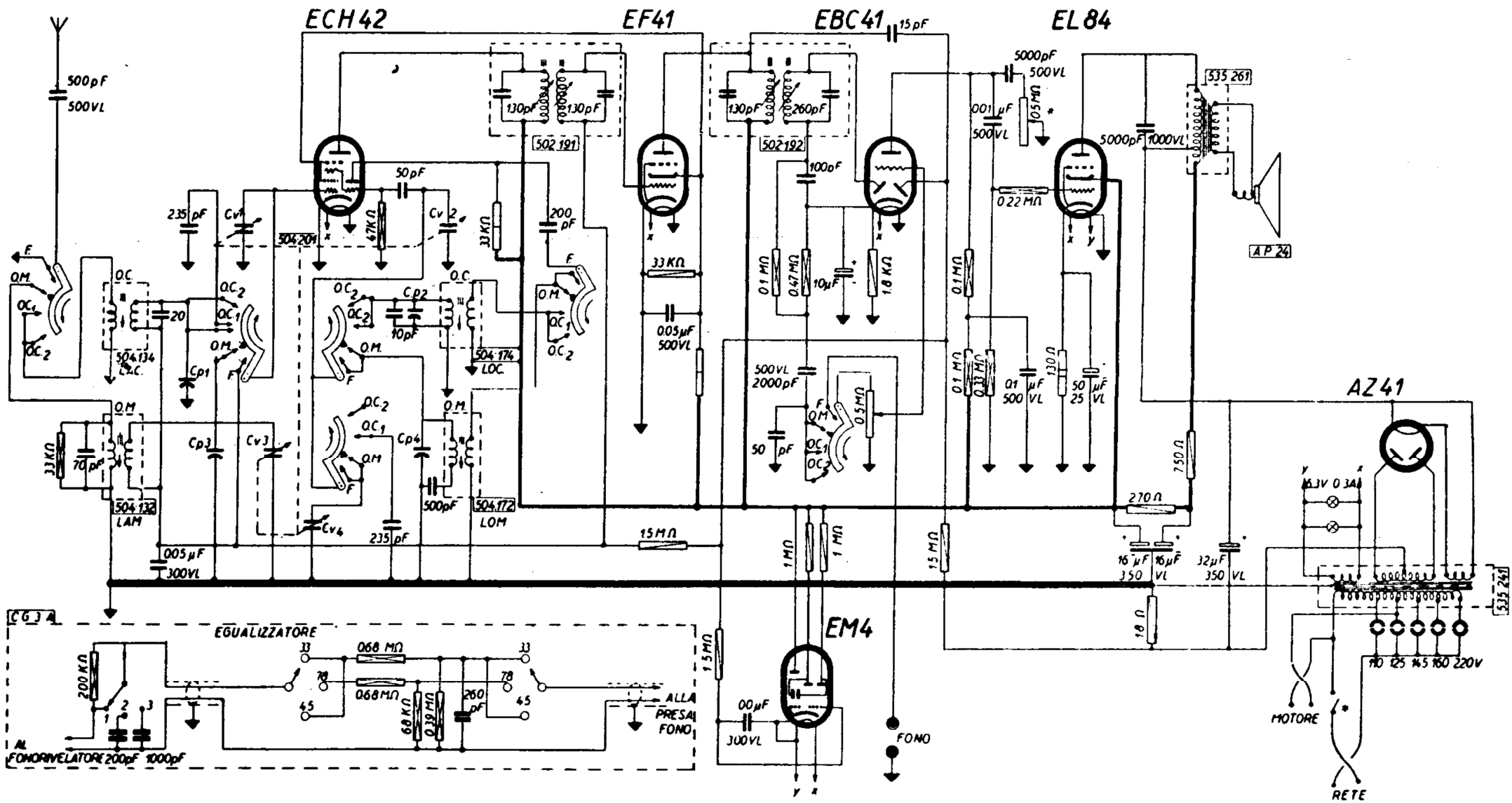
VOCE DEL PADRONE - FONORADIO mod. 535. Onde medie e 2 gamme espanse onde corte. Media frequenza 465 kc/s. Potenza indistorta di uscita 4 watt. Consumo 60 watt.
